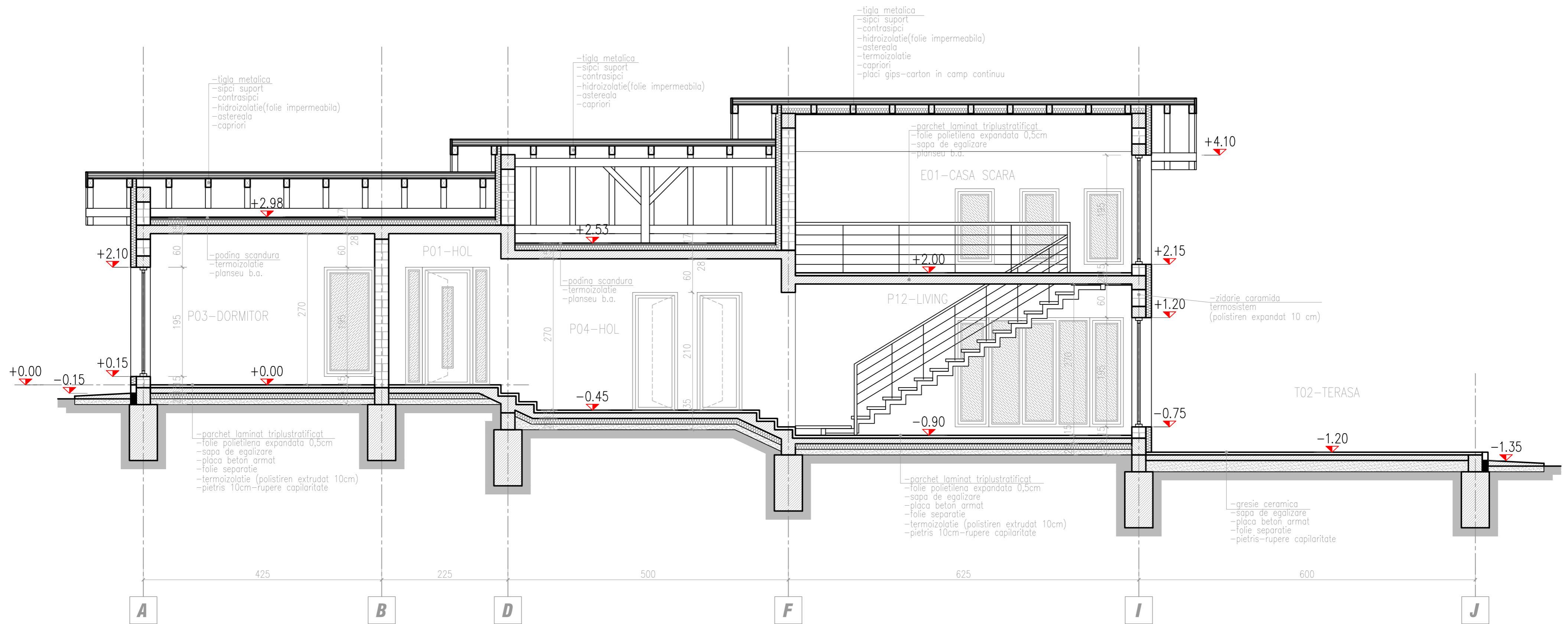
SECTIUNE A-A
